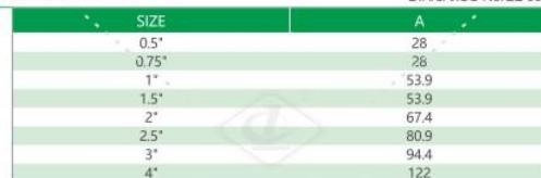
DIN/3A/ISO No.QL-006
