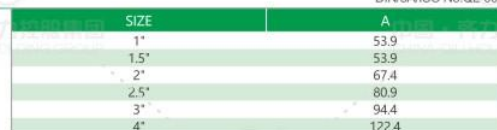
DIN/3A/ISO No.QL-004
