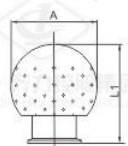
卡箍式固定式清洗球 Clamp static cleaning ball
