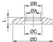
快装盲板 Bored Flange
