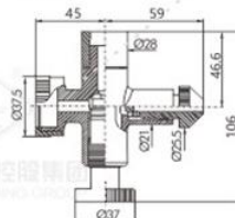
液位计 Liquidometer
