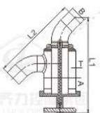
Y型过滤器 Y-type filter
