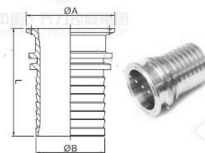
卡盘软管接头 Clamp Hose Adapter
