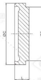
DIN/ISO/IMPERIAL - 14 LINER BLANK CAP
