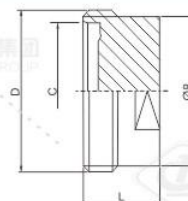
DIN/ISO/IMPERIAL - 14 LINER BLANK CAP
