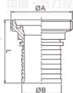
DIN软管接头 DIN hose adapter
