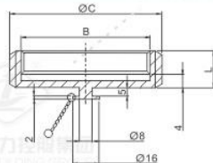
SMS-13R RBN BLANK NUT
