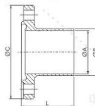
IMP ERIAL Nutflansch(NF)
